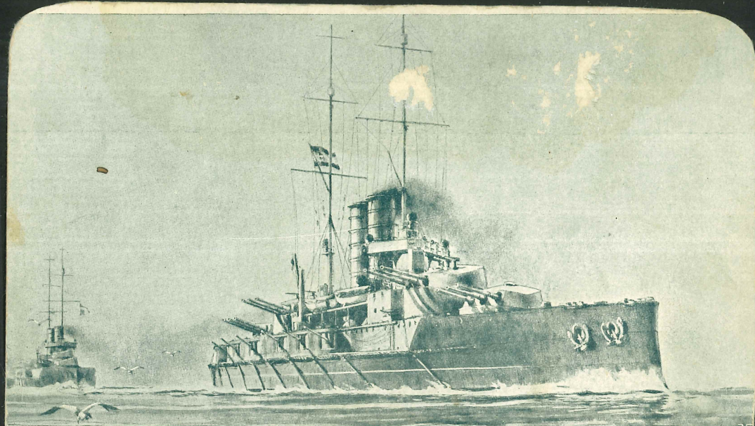
Австро-Венгрия. Дредноутъ Viribus Unitis 20.300 т. 1911 г. 20,8 узловъ. Артиллерія: XII—12 дм., XII—6 дм., XVIII—3 дм., II—мелк.
